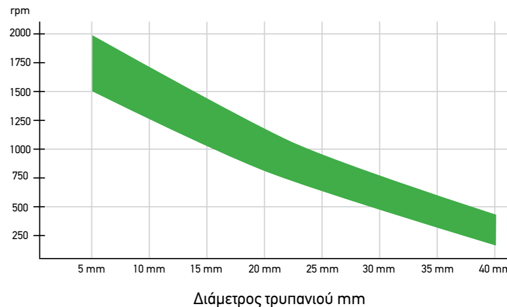
Εύρος βέλτιστης ταχύτητας διάτρησης σε rpm (στροφές ανά λεπτό)
